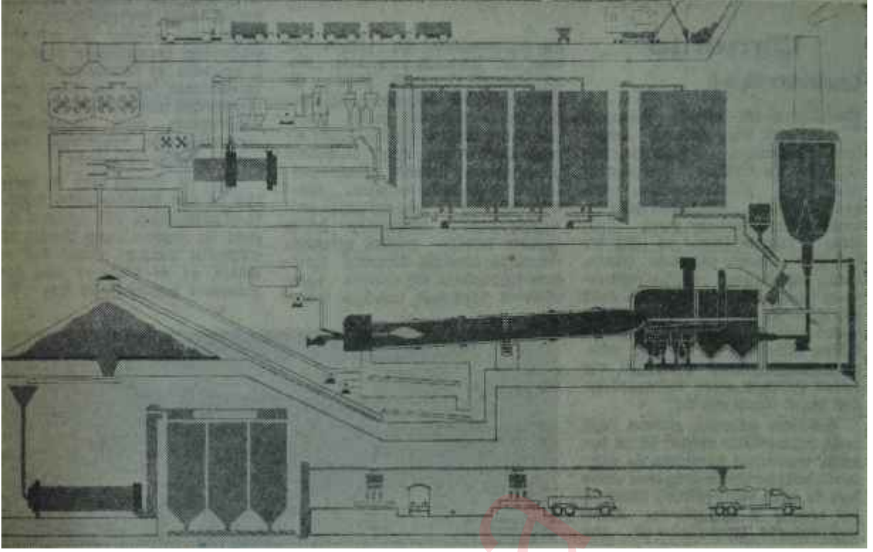
Kuru usulde çimento imali şeması
