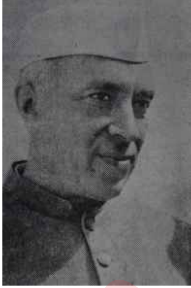
Nehru
