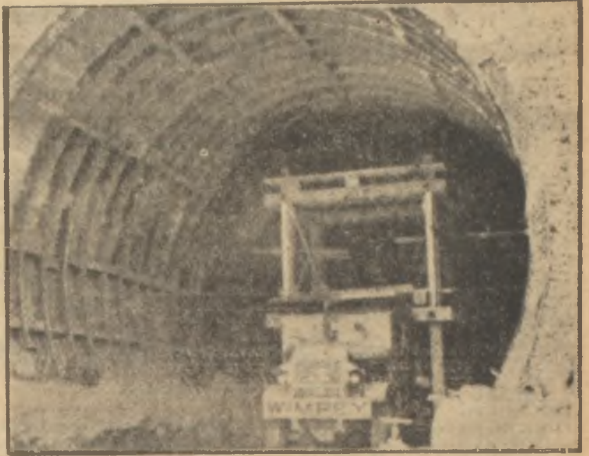
Hırfanlı Barajının tünelinin ağzı
